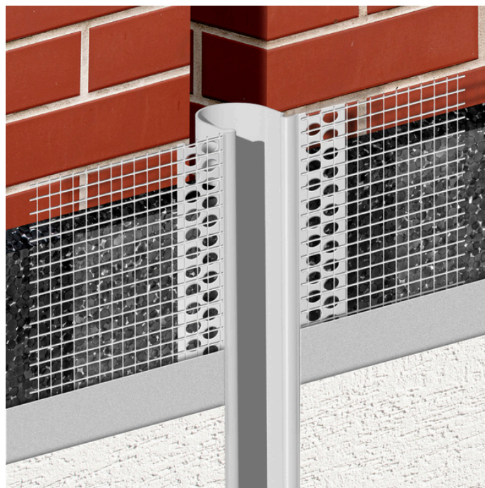
Grafika użytkowa do stosowania produktu PVC PROFIL DYŁ P.
